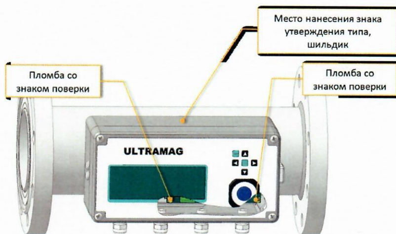
Рисунок 3 – Схема пломбировки комплекса с фланцевым присоединением (базовый ИВБ), указание места нанесения знака утверждения типа, расположение шильдика
